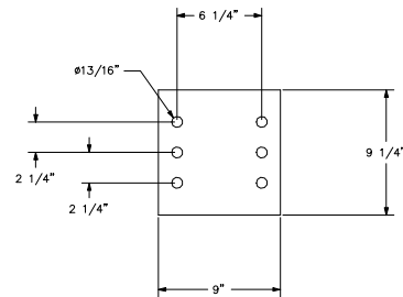
DETAIL A-A (TYP)
